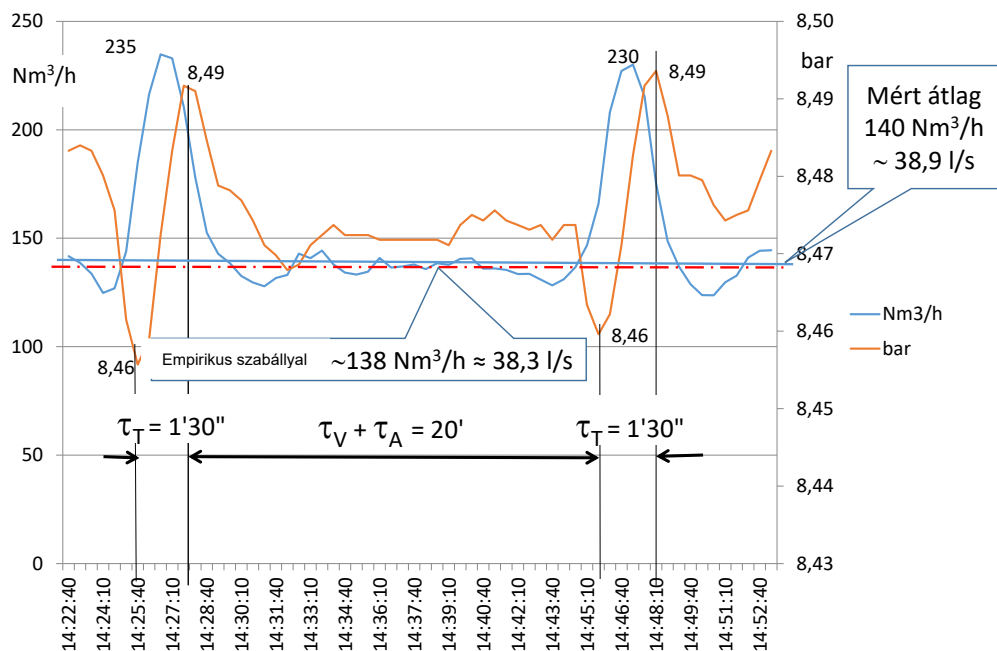
1.1.5.1. ábra Sűrített levegő hálózat nyomás-, levegőáram- és szivárgás-diagramja a mérendő periódusidők feltüntetésével
