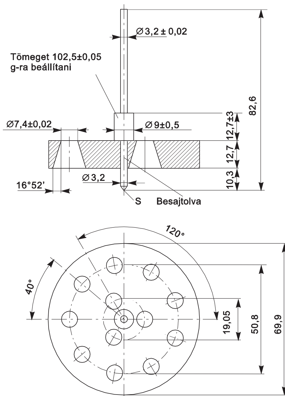
4. ábra: Penetrométer
